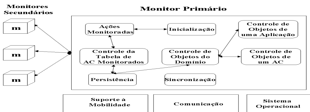
Figura 5. Apresentação da arquitetura em módulos do monitor primário.
