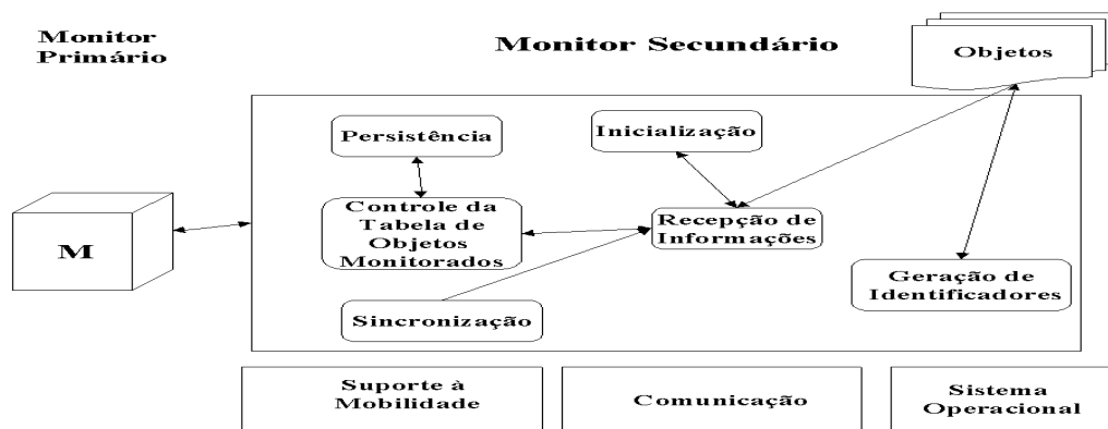
Figura 6. Apresentação da arquitetura em módulos do monitor secundário.
