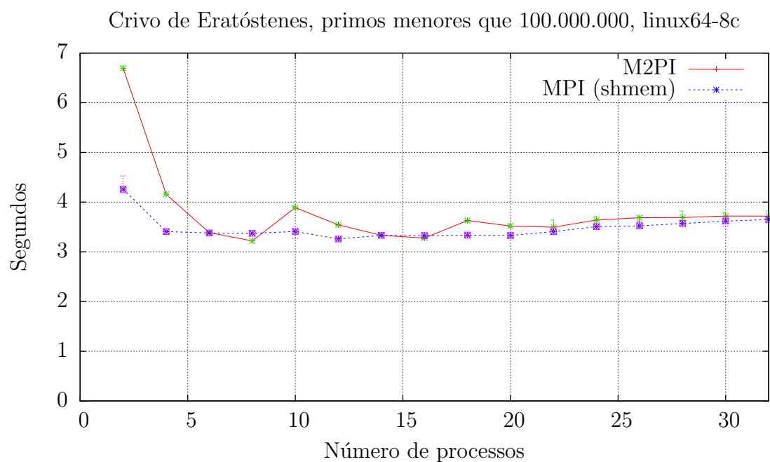
Figura 7.4: CE variando o número de processos
