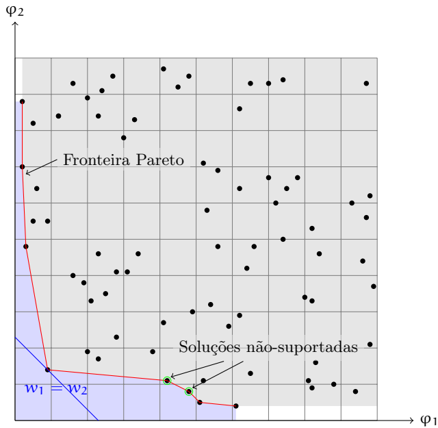
Figura 5.2.: Soluções de um problema com duas funções objetivo. Fronteira eficiente em vermelho. A solução ótima ponderada com pesos w_1 = w_2 em azul. Duas soluções eficientes não-suportadas marcadas em verde.
