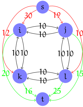
Figura 1.10: Exemplo da construção para uma imagem 2 \times 2 . Direita: Tabela com valores pele/não-pele. Esquerda: Grafo com penalidade fixa p_{ij} = 10 .
