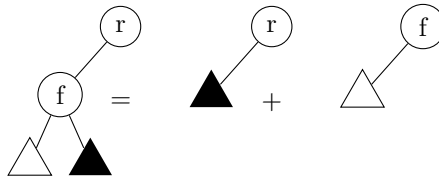
Figura 1.4: Separar uma semi-árvore de posto k em duas.
