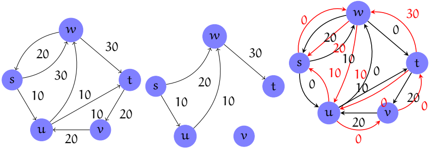
Figura 1.6: Esquerda: Grafo com capacidades. Centro: Fluxo com valor 30. Direita: O grafo residual correspondente.
