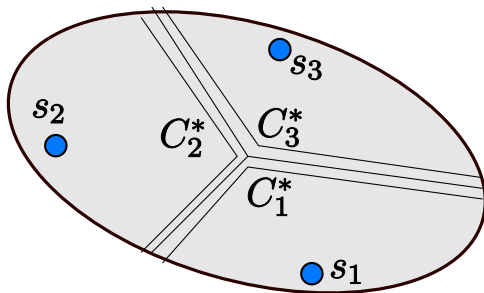
Figura 3.4.: Corte múltiplo e decomposição em cortes isolantes.
