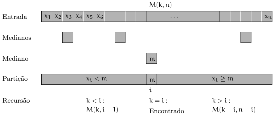
Figura A.1.: Funcionamento do algoritmo recursivo para seleção.
